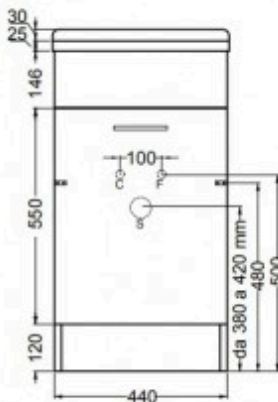
VISTA FRONTALE
