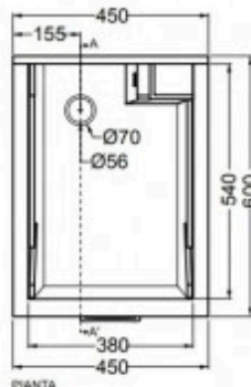
PIANTA
