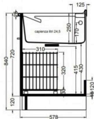
SEZIONE A-A'
